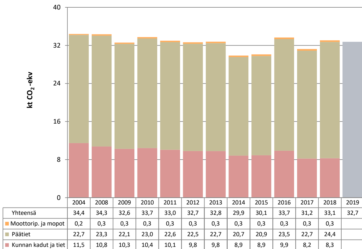
Kuva 8. Tieliikenteen päästöt Ylivieskassa vuonna 2004 ja vuosina 2008–2019. Vuoden 2019 tieto on ennakkotieto, joka perustuu liikennemäärien muutoksiin kunnan alueella.
