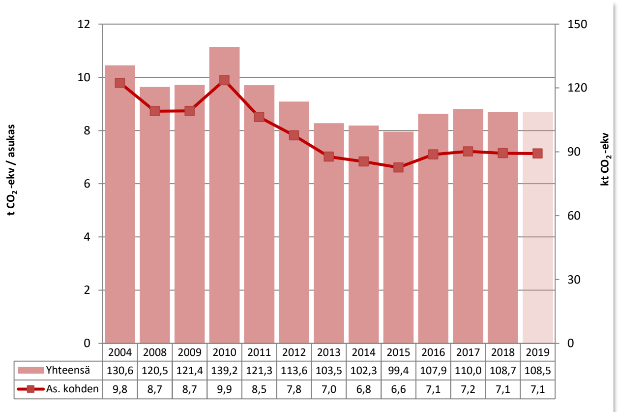
Kuva 17. Päästöt yhteensä ja asukasta kohden Ylivieskassa vuonna 2004 ja vuosina 2008–2019 ilman teollisuutta. Vuoden 2019 tieto on ennakkotieto.
