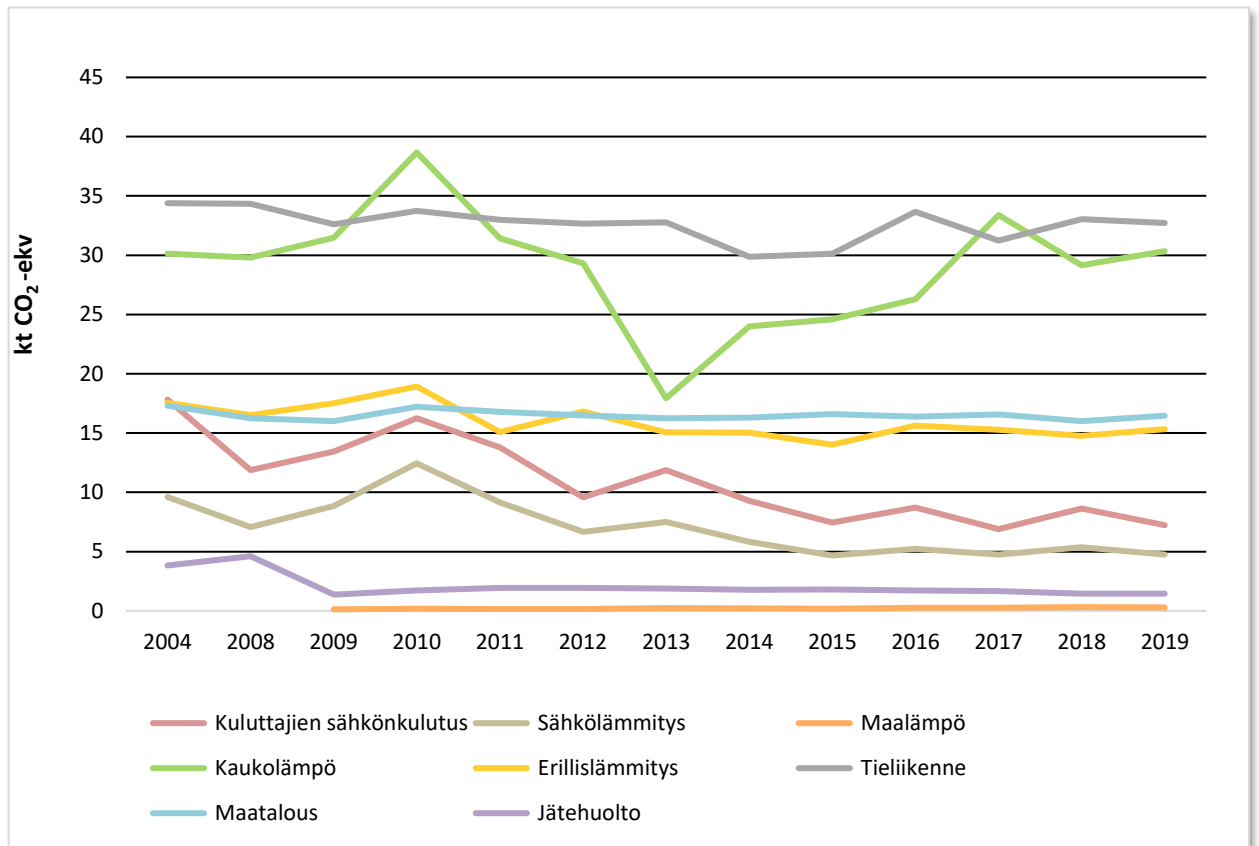
Kuva 16. Sektorikohtaisten päästöjen kehitys Ylivieskassa vuonna 2004 ja vuosina 2008–2019. Vuoden 2019 tiedot perustuvat osittain ennakkotietoihin.
