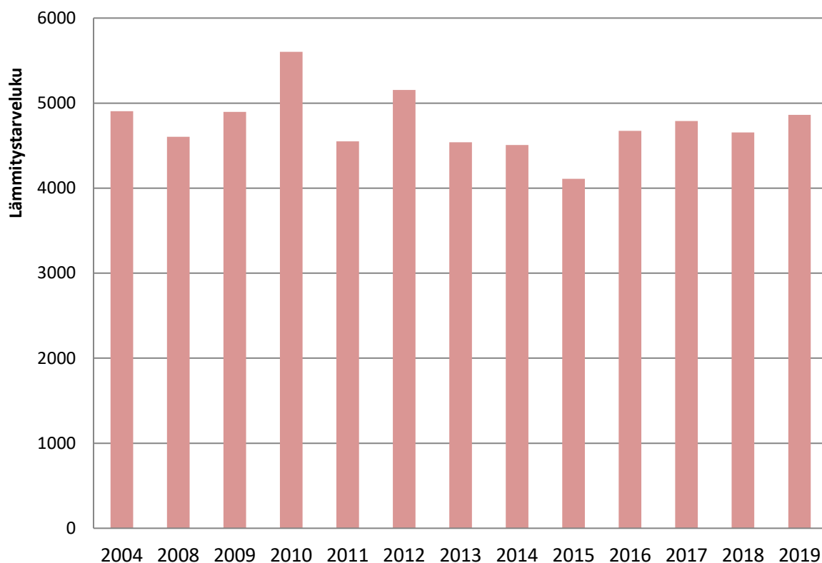
Kuva 4. Ylivieskan lämmitystarveluvut vuonna 2004 ja vuosina 2008–2019.
