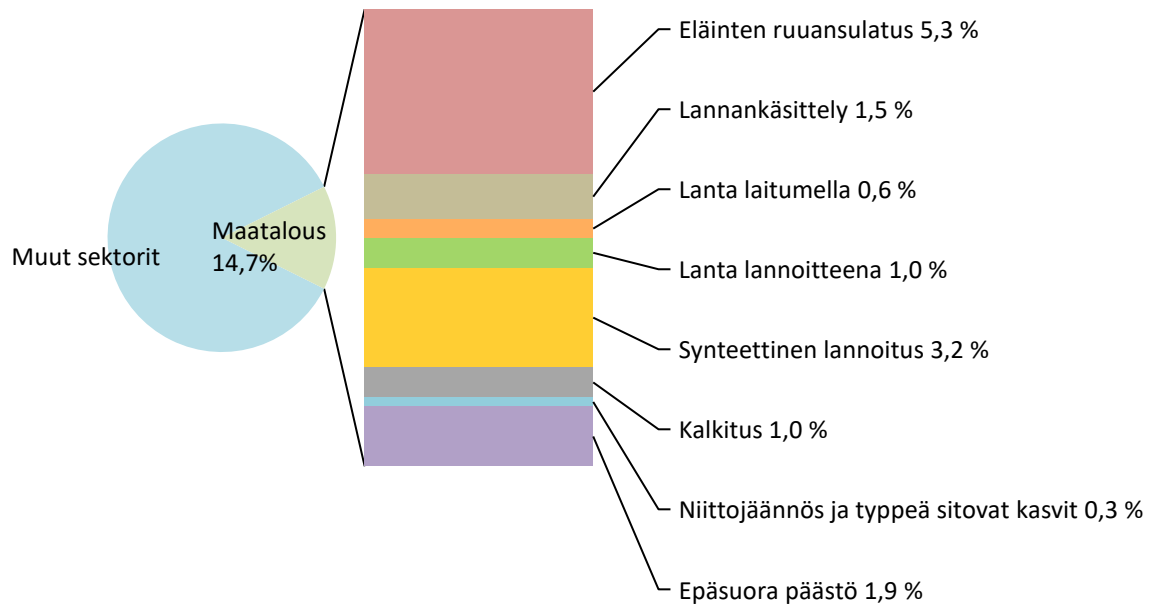
Kuva 9. Maatalouden päästöjen osuus kokonaispäästöistä (ilman teollisuutta) Ylivieskassa vuonna 2018 ja sektorin jakautuminen eri päästölähteisiin.
