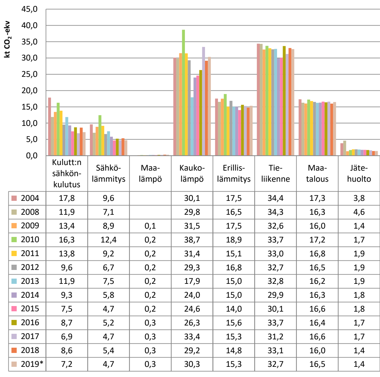
Kuva 15. Päästöt sektoreittain Ylivieskassa vuonna 2004 ja vuosina 2008–2019 ilman teollisuutta. Vuoden 2019 tieto on ennakkotieto.
