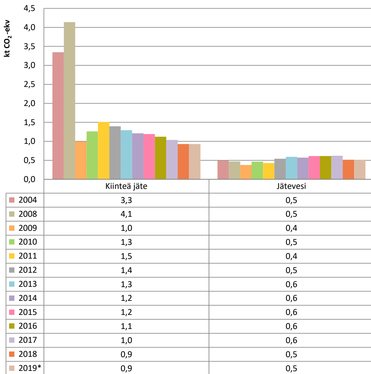
Kuva 12. Jätehuollon päästöjen kehitys Ylivieskassa vuonna 2004 ja vuosina 2008–2019. Vuoden 2019 ennakkotietona on vuoden 2018 tieto.
