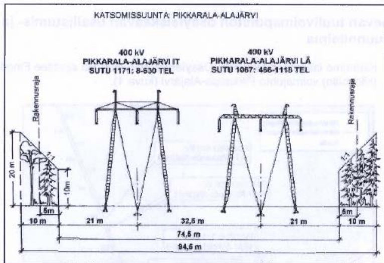
Kuva 2. Fingridin 2x400 kV voimajohdon poikkileikkaus.
