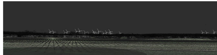
Kuva 645 (3d-rautalankamalli, pistepilvi)
